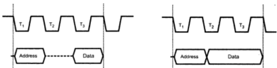
Fig. 1.24 Data bus
